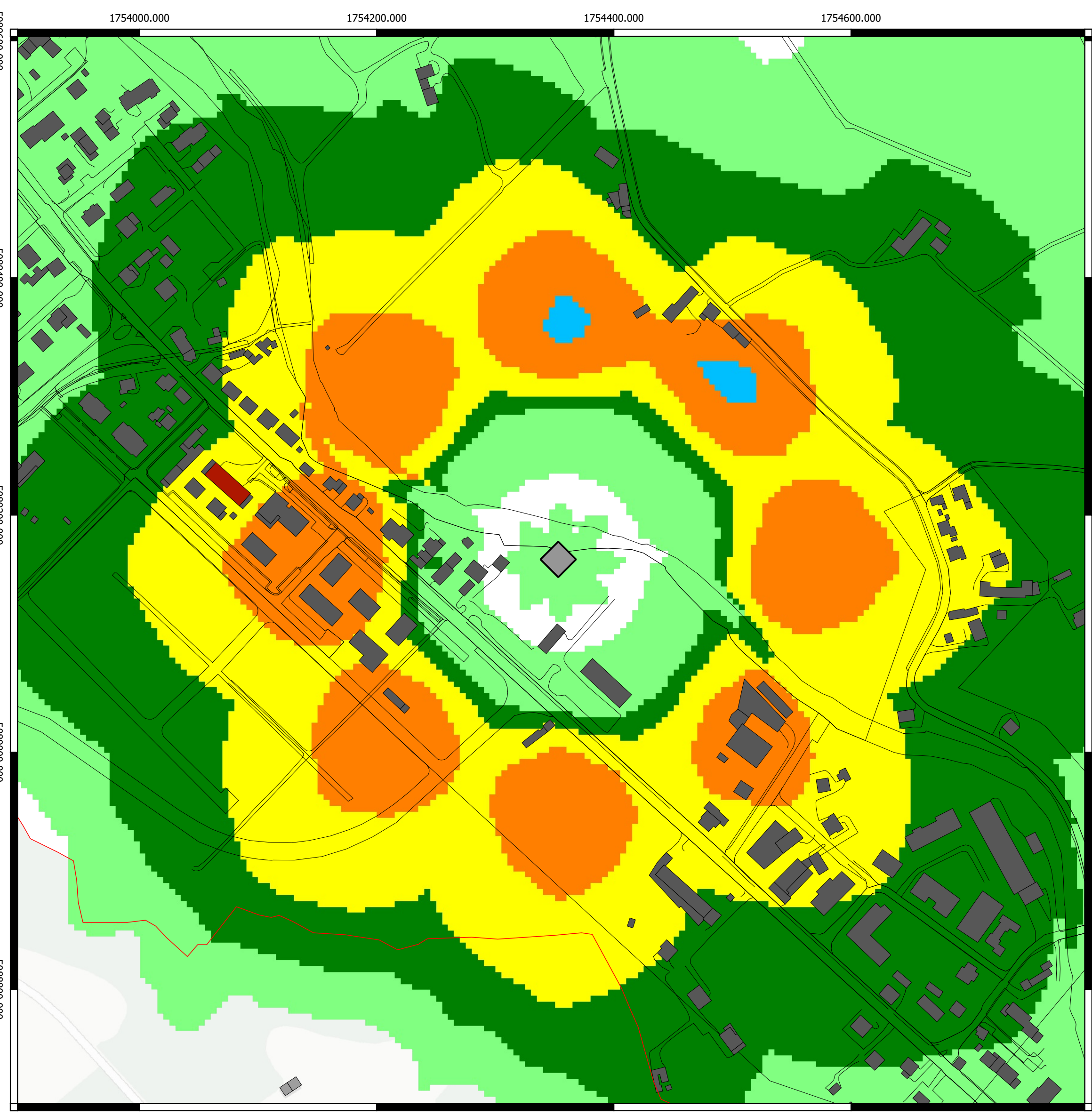
Campo elettromagnetico (V/m) calcolato alla quota di 11,5 m sul livello del terreno
